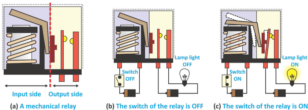
Fig. 17.10: Relay
