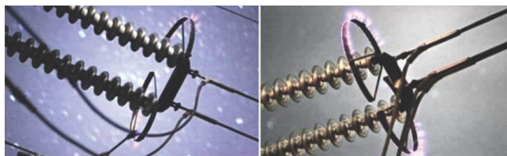
Fig. 15.17: Corona discharge
